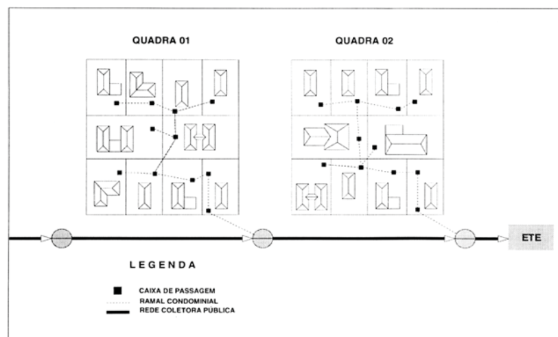
Figura 9 - Modelo físico de sistema condominial. Fonte: SPERLING; COSTA; CASTRO (1995, p.138)
