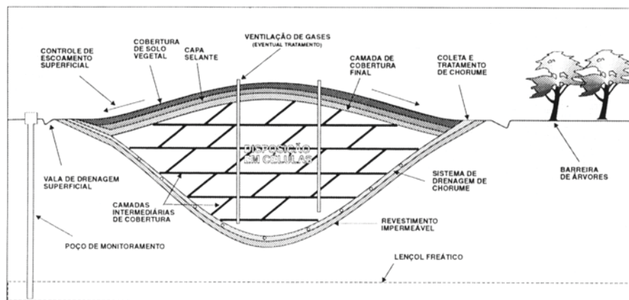
Figura 1 - Corte esquemático de um aterro sanitário.
