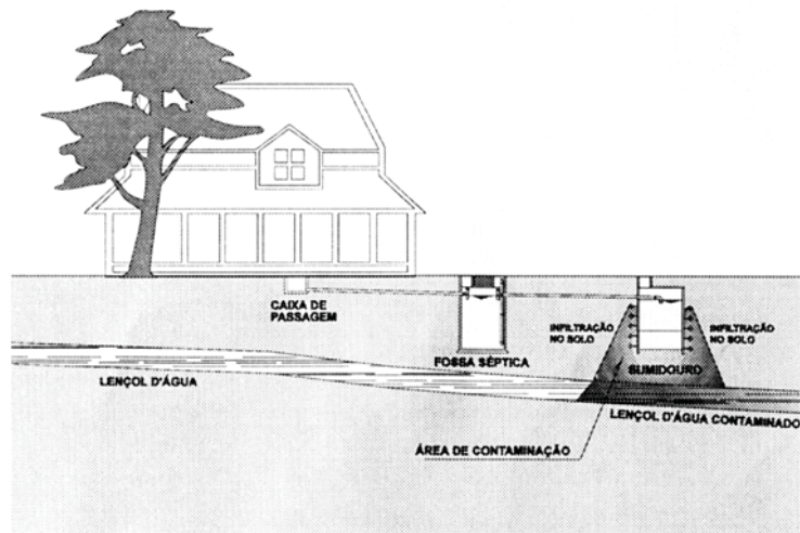
Figura 5 - Riscos de contaminação da água subterrânea pelos esgotos. Fonte: SPERLING; COSTA; CASTRO (1995, p.123)
