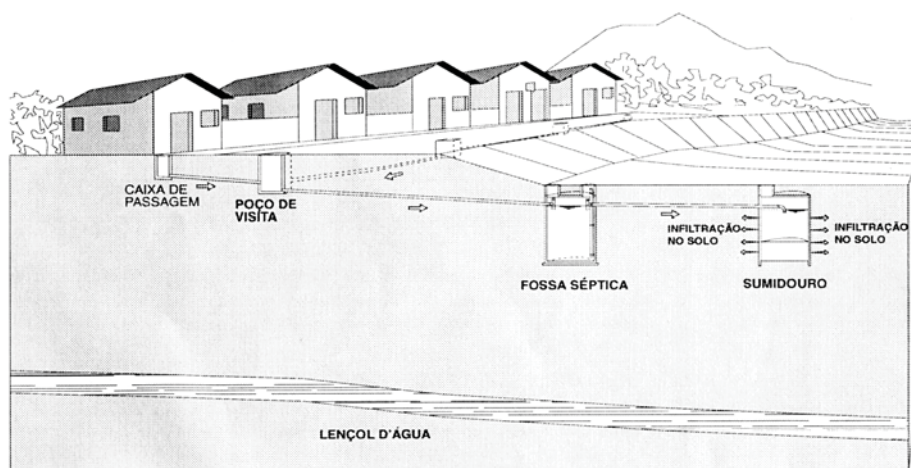
Figura 6 - Fossa séptica como solução coletiva. Fonte: SPERLING; COSTA; CASTRO (1995, p.124)
