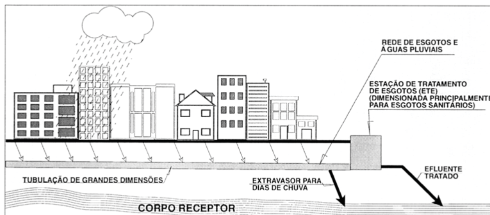
Figura 7 - Sistema unitário ou combinado. Fonte: SPERLING; COSTA; CASTRO (1995, p.125)
