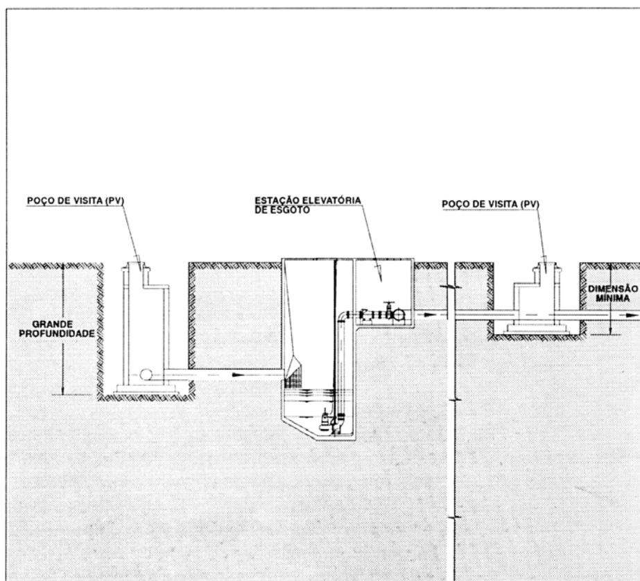
Figura 10 - Estações elevatórias. Fonte: SPERLING; COSTA; CASTRO (1995, p.139)
