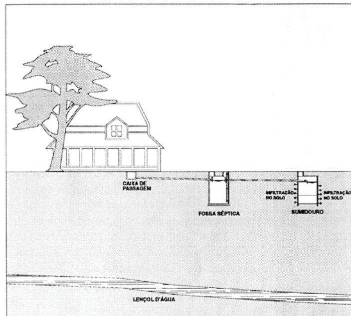
Figura 4 - Solução Individual. Fonte: SPERLING; COSTA; CASTRO (1995, p.123)
