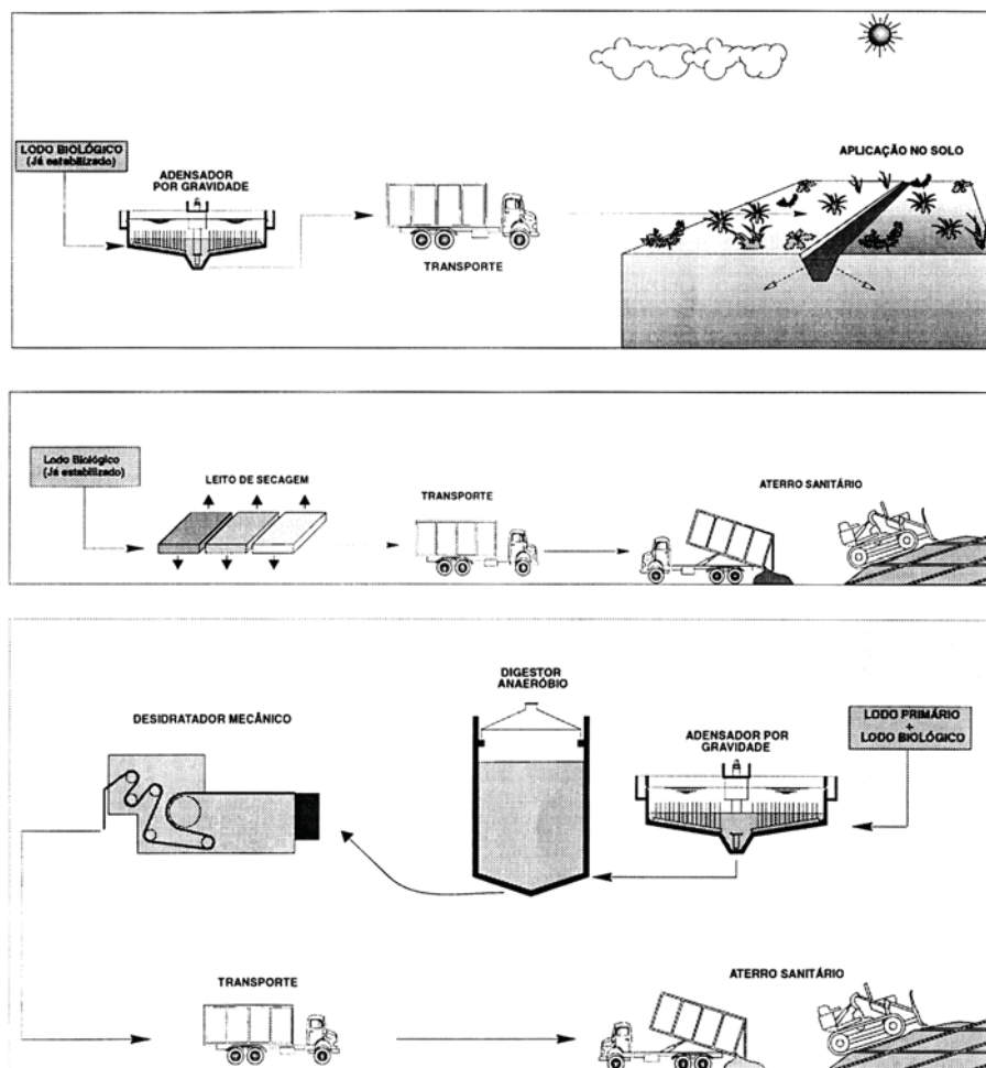
Figura 12 – Algumas alternativas de tratamento e disposição do lodo. Fonte: SPERLING; COSTA; CASTRO (1995, p.155)
