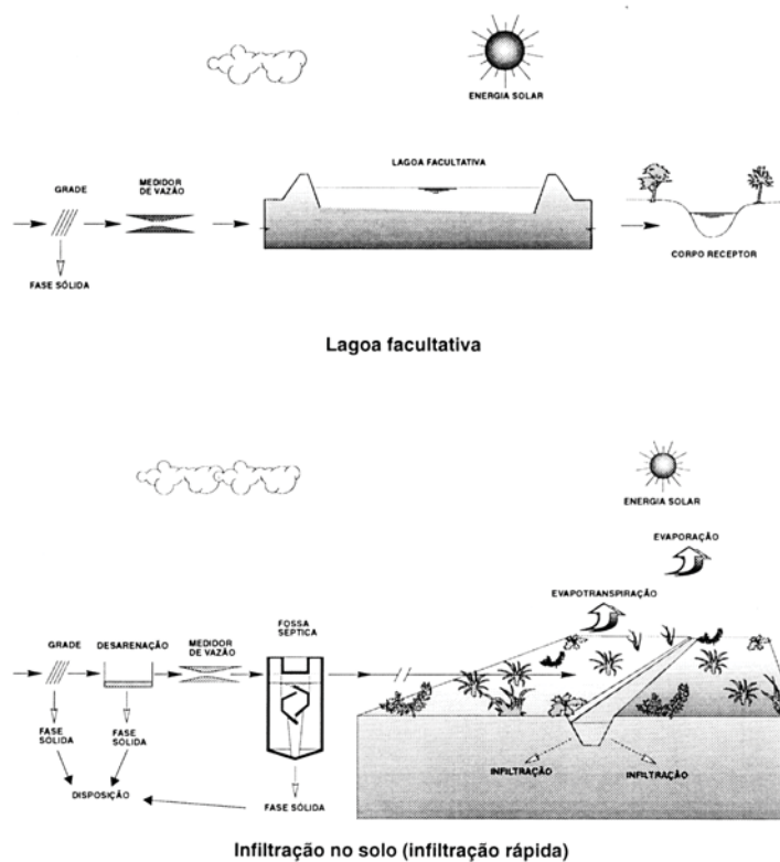
Figura 11 – Lagoa Facultativa e a Infiltração rápida no solo. Fonte: SPERLING; COSTA; CASTRO (1995, p.149)
