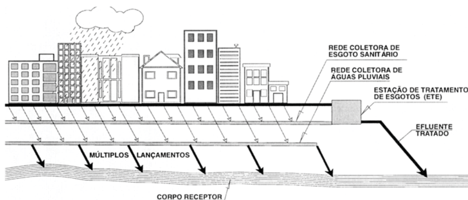
Figura 8 - Sistema separador. Fonte: SPERLING; COSTA; CASTRO (1995, p.126)
